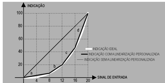
Figura 2 – Um sinal não linear submetido a uma linearização personalizada.
