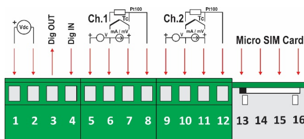
Fig. 42 – Conexões Elétricas
