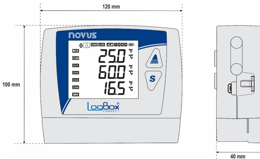
Fig. 37 – Dimensões do LogBox 3G
