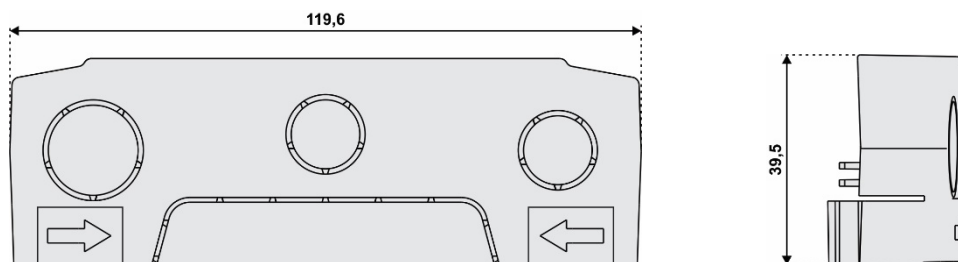
Fig. 34 – Dimensões da Tampa de Proteção das Conexões e Cavidades Destacáveis
