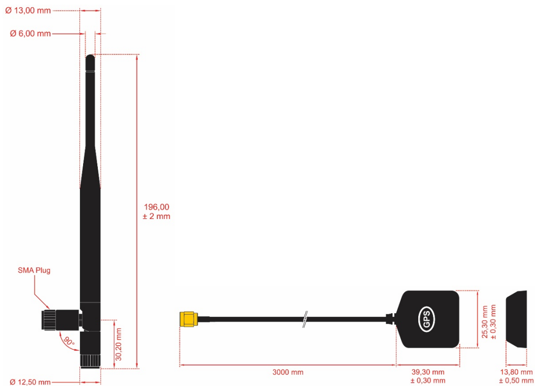
Fig. 38 – Dimensões das antenas (celular e GPS)
