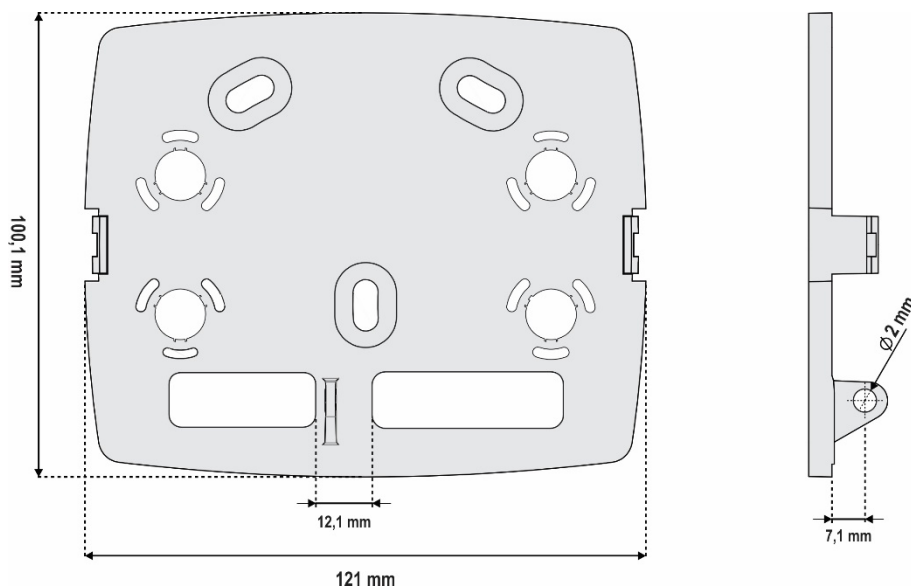
Fig. 32 – Suporte de Fixação
