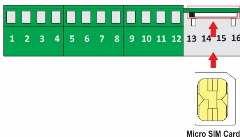
Fig. 41 – Conexão Micro SIM Card
