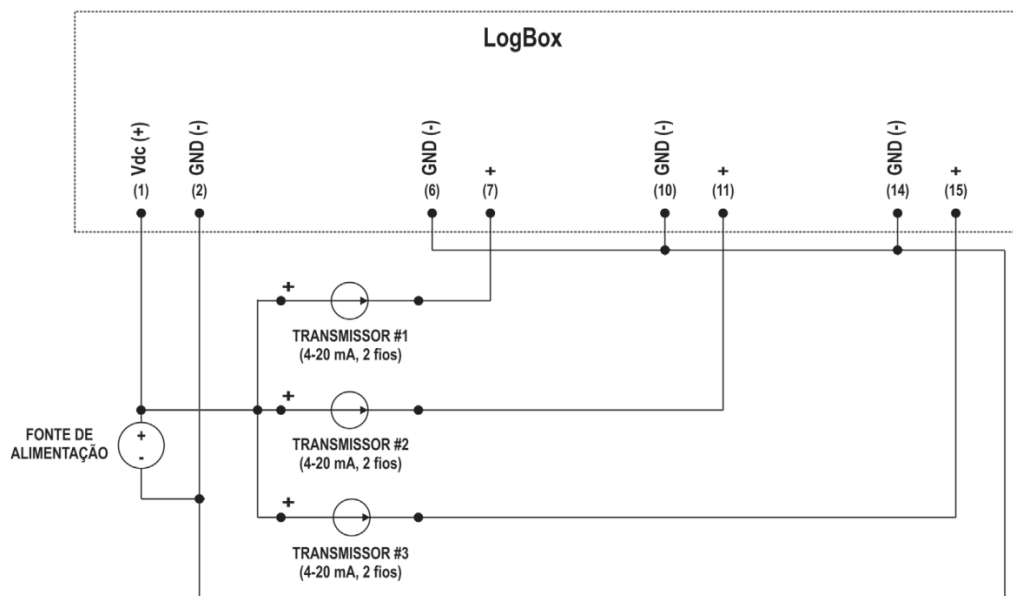
Fig. 43 – Exemplo de ligação de transmissores alimentados pelo loop
