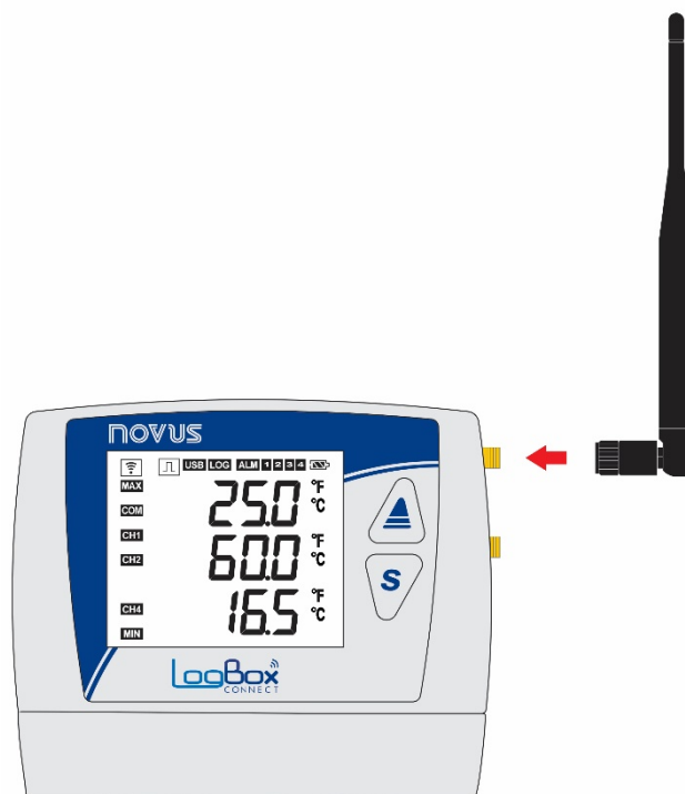
Fig. 39 – Antena de telefonia celular
