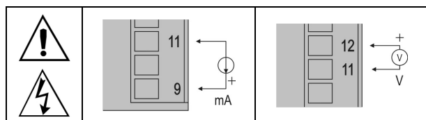
Figura 03 - Conexões de sinais de corrente (mA) e tensão (V)
