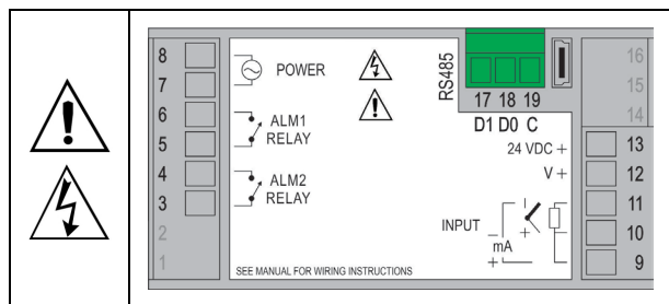
Figura 01 – Painel traseiro do indicador
