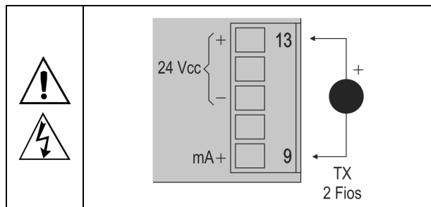
Figura 04 – Exemplo de utilização da fonte de tensão auxiliar do indicador
