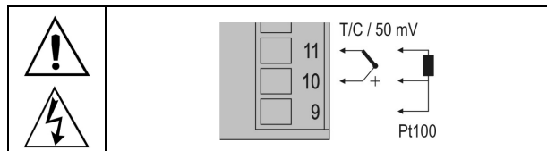
Figura 02 - Conexões de Pt100 três fios, Termopares e sinal de 50 mV
